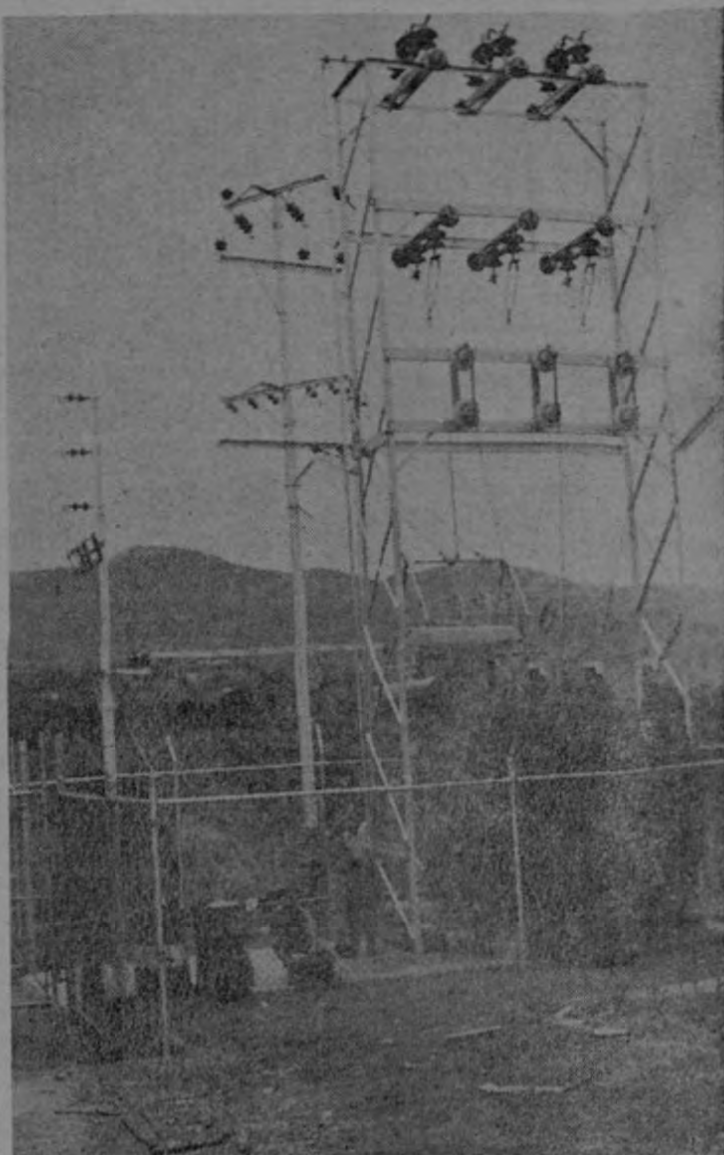
Aspecto general de la nueva y moderna subestación que instaló la Compañía Nacional de Fuerza y Luz, S. A. en Anonos, por financiamiento de la Caja Costarricense de Seguro Social, para suministrar mejores servicios y atender el aumento en la demanda de carga, entre sectores importantes: Las Pavas, Anonos y La Sabana.
