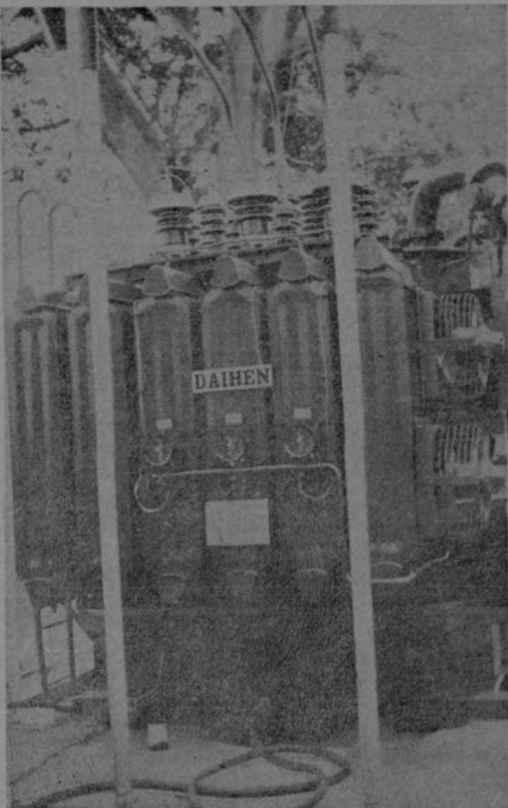
Moderna subestación con capacidad de 14,000 K.V.A., instalada en los terrenos de la Planta Anonos, para mejorar los servicios a Las Pavas, La Sabana y Anonos, debido al notable crecimiento de población industrial y residencial de esos lugares. Esta obra fue financiada por la Caja Costarricense de Seguro Social.
